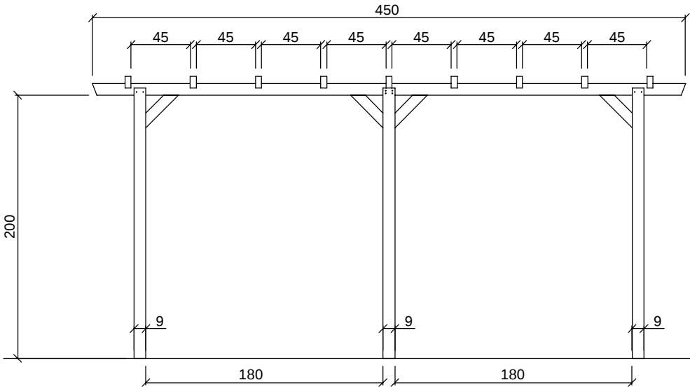
Vorderansicht
