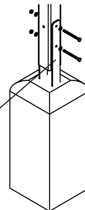
Pfostenträger
