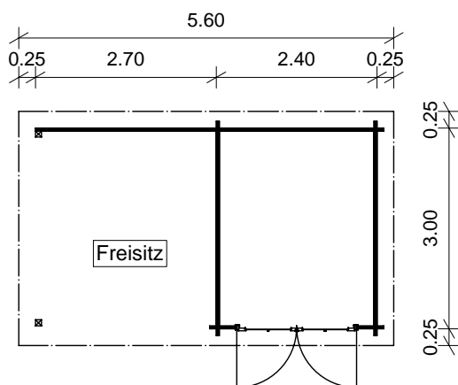
Grundriß
