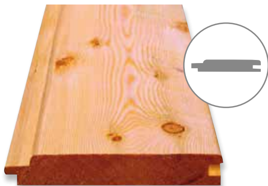
Rundkantenprofil im Schnitt: 19,5 x 96 mm mit Nut und Feder. Bsp. zeigt „Natur“ (Lärche).
