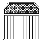
Zaunfeld mit Rankgitter, beidseitig abgeschrägt B 1.800 x 1.800/1.500 mm
