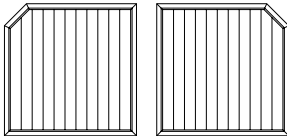
Zaunfeld geschlossen, einseitig abgeschrägt, links/rechts B 1.800 x 1.800/1.500 mm
